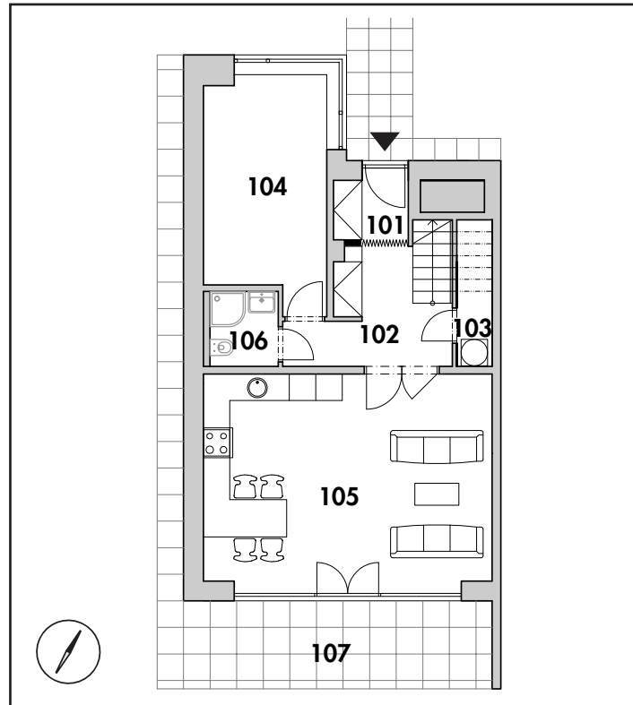
1. NP Púdorys ▼
