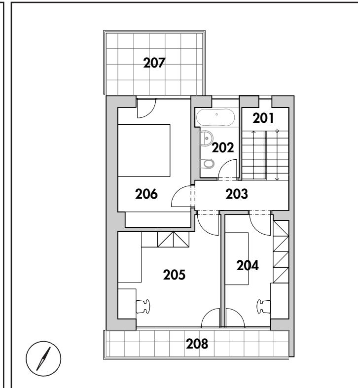
2. NP Púdorys ▼
